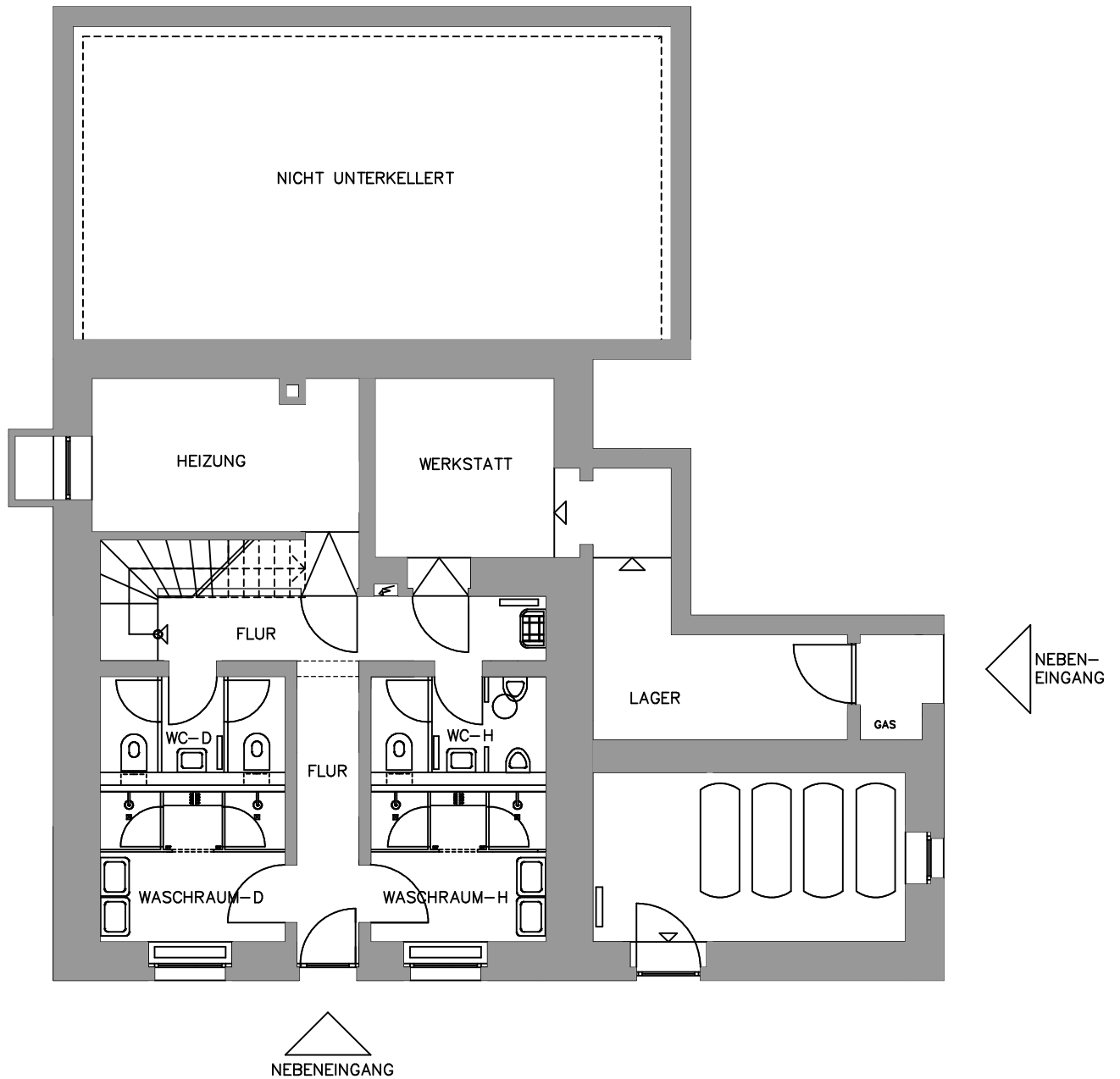
UNTERGESCHOSS – SCHWARZSCHNIEDERHOF
